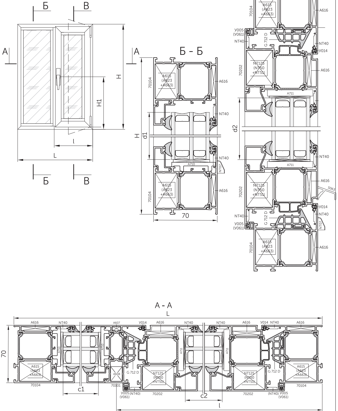
Тип X - вариант комбинированного окна Вид со стороны помещения
