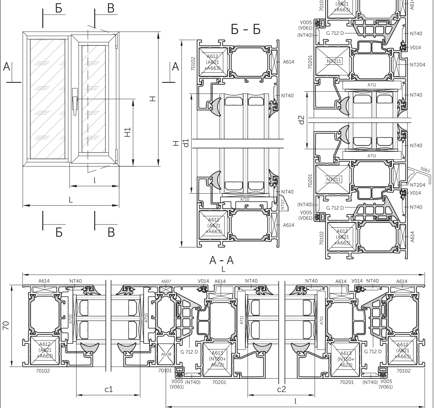
Тип VII - вариант комбинированного окна Вид со стороны помещения
